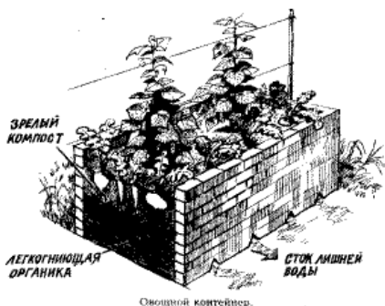
Овощной контейнер.
